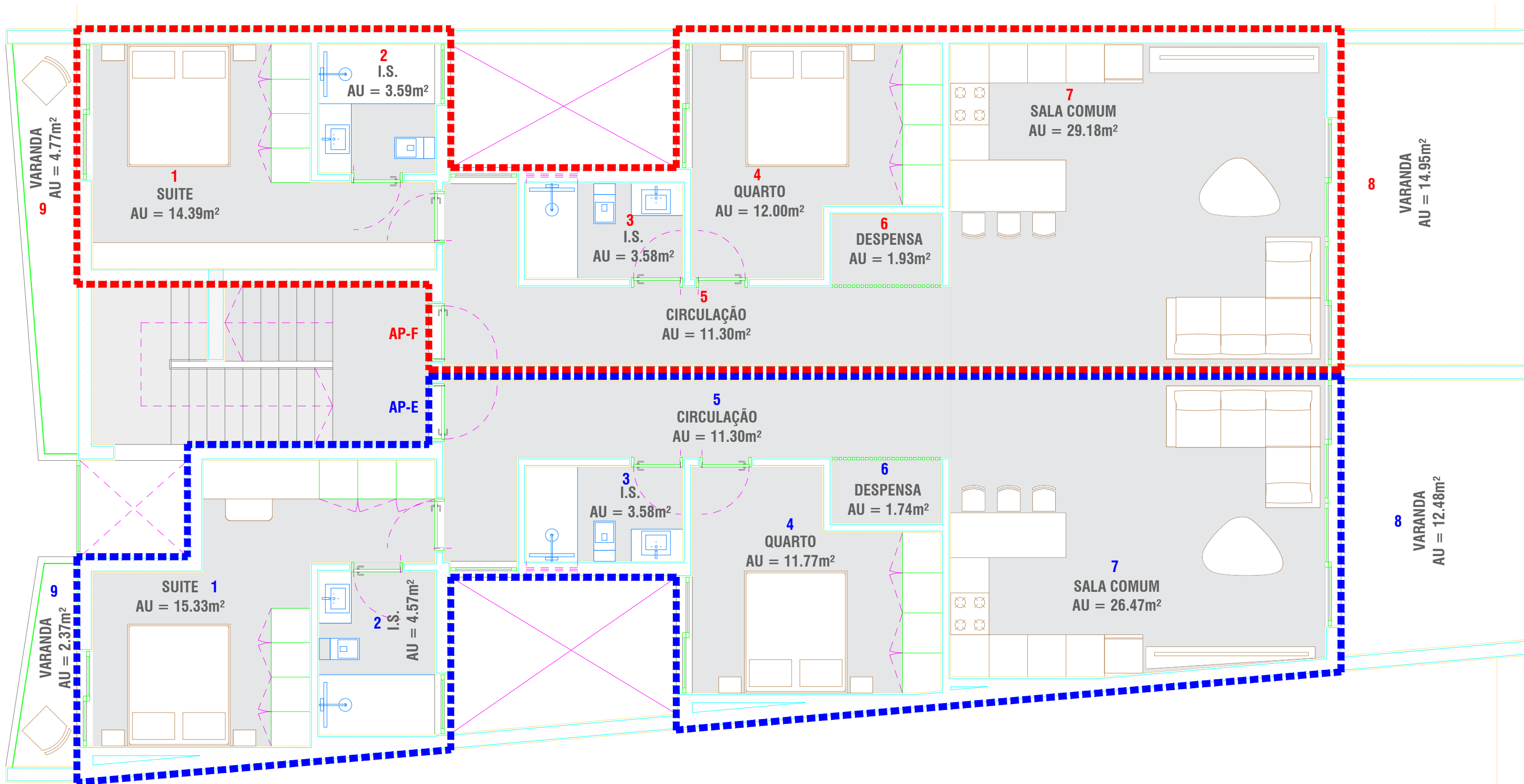
PLANTA_2º ANDAR
