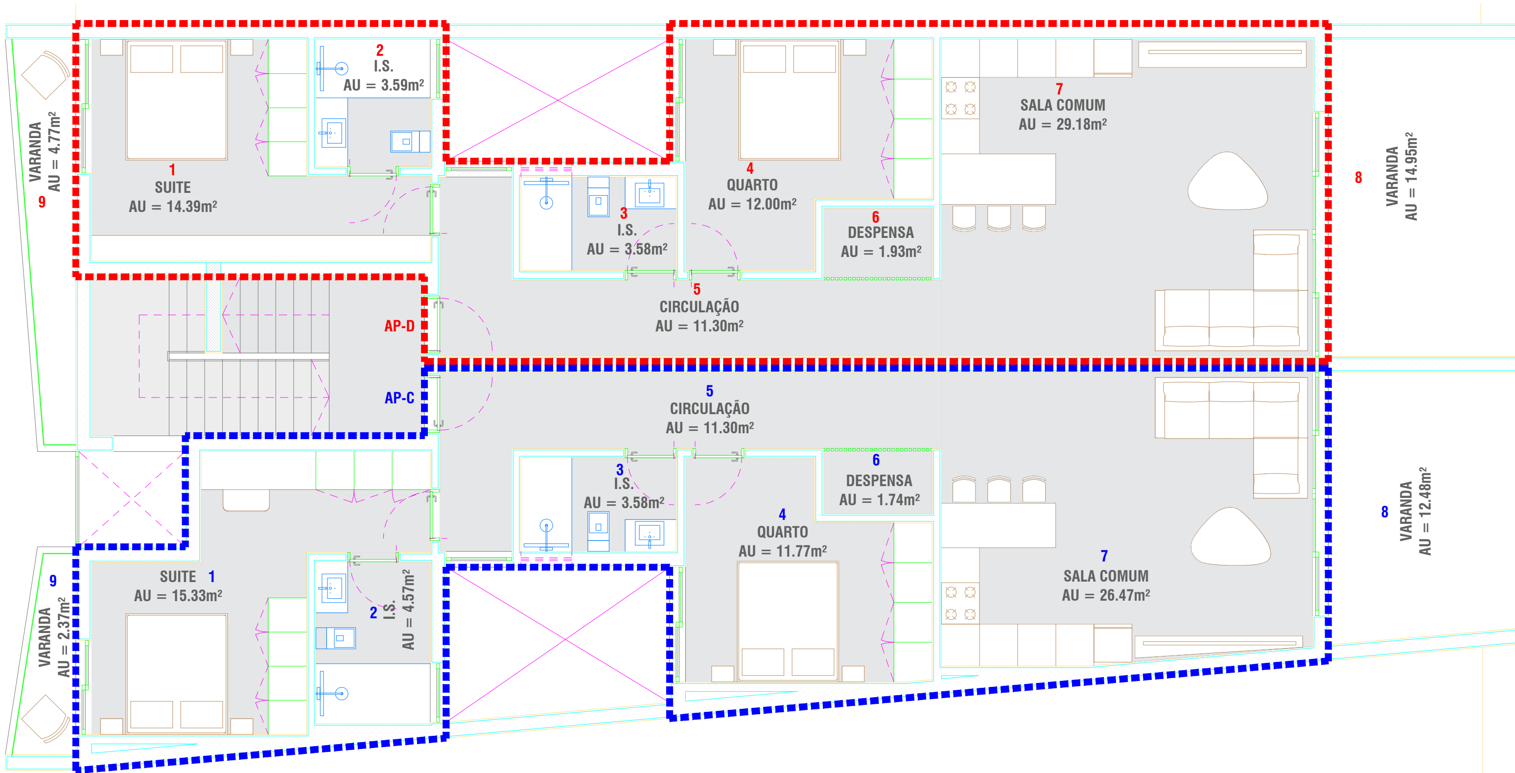
PLANTA_1º ANDAR
